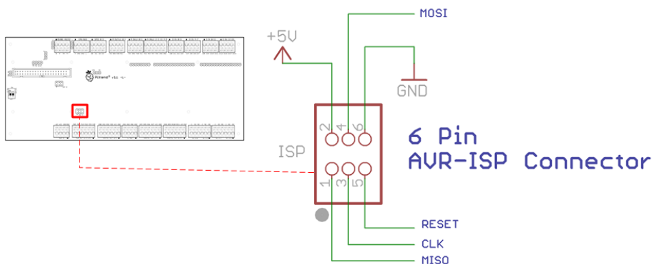
Abbildung 57: Prinzip-Schaltbild: Anschluss eines Programmieradapters an ISP 1 - ATtiny441
