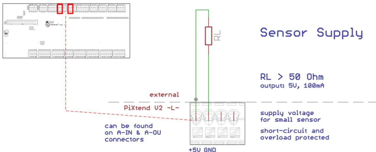
Abbildung 72: Prinzip-Schaltbild: Anschluss der Sensorversorgung
