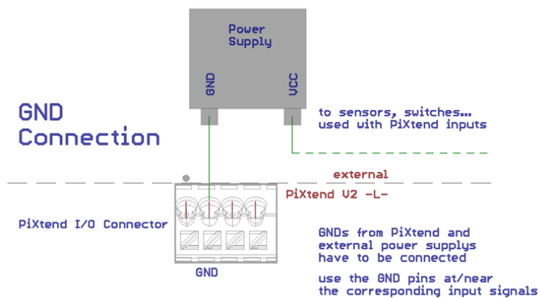
Abbildung 73: Prinzip-Schaltbild: GND-Verbindung
