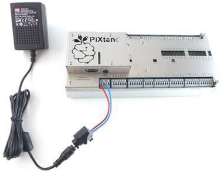
Abbildung 40: Anschluss des Netzteils an PiXtend V2 -L-
