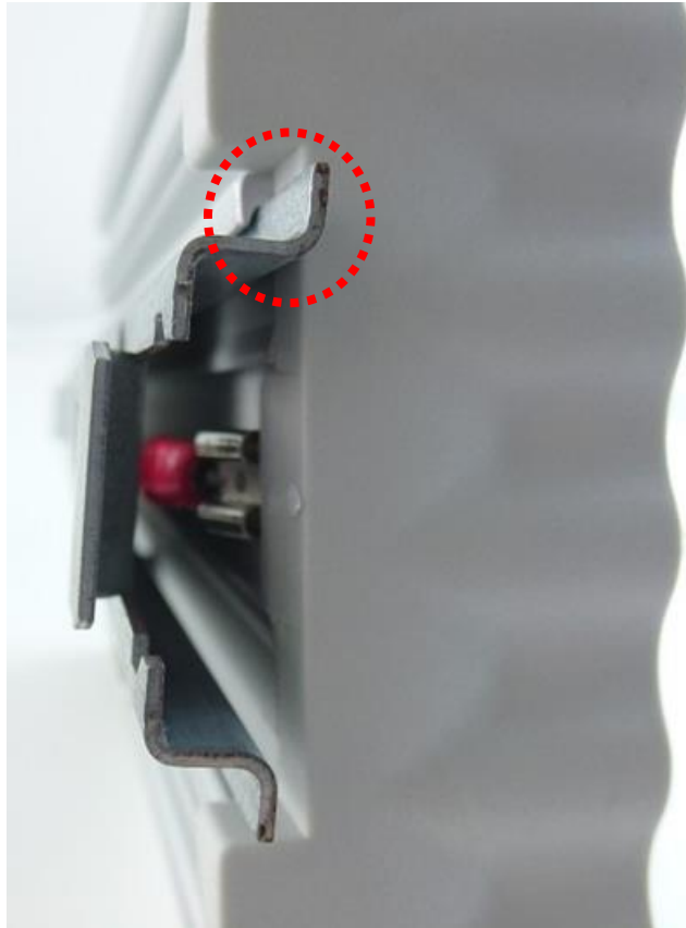
Abbildung 17: Gehäuse auf Hutschiene eingehängen
