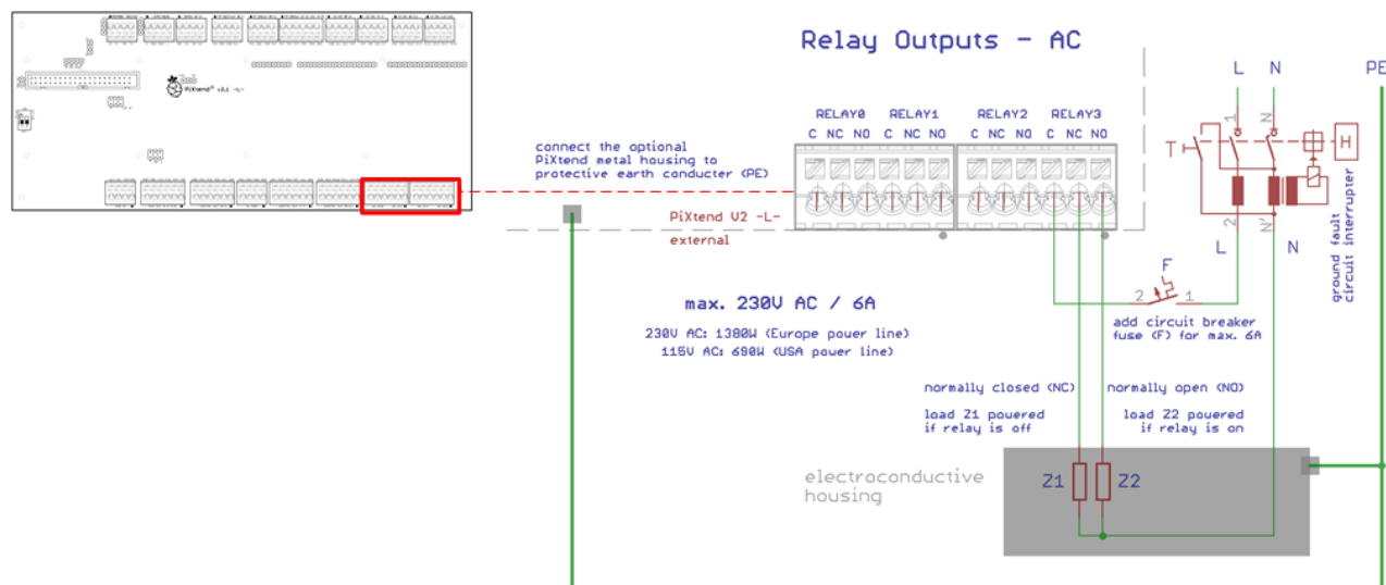
Abbildung 65: Prinzip-Schaltbild: Anschluss der Relais (Wechselspannung)
