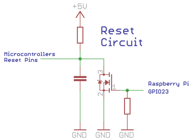
Abbildung 54: Prinzip-Schaltbild: Reset-Schaltung
