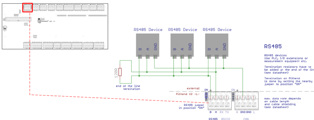
Abbildung 83: Prinzip-Schaltbild: Anschluss der RS485-Schnittstelle
