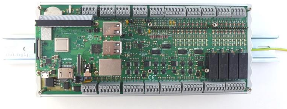
Abbildung 18: Hutschienenmontage abgeschlossen
