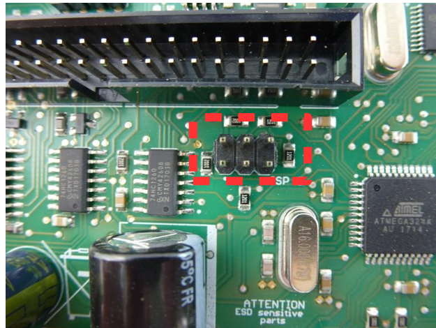
Abbildung 52: ISP 0 Steckverbinder - In-System-Programmierung (ISP) - ATmega324A
