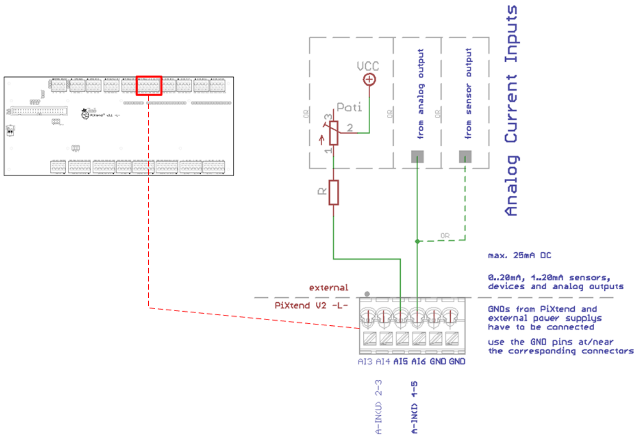
Abbildung 74: Prinzip-Schaltbild: Anschluss der analogen Stromeingänge
