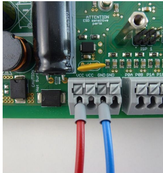
Abbildung 39: Versorgungsanschluss auf PiXtend V2 -L-
