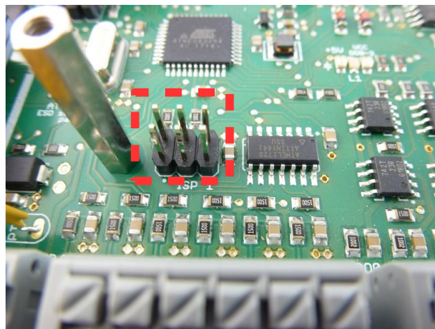
Abbildung 53: ISP 1 Steckverbinder - In-System-Programmierung (ISP) - ATtiny441
