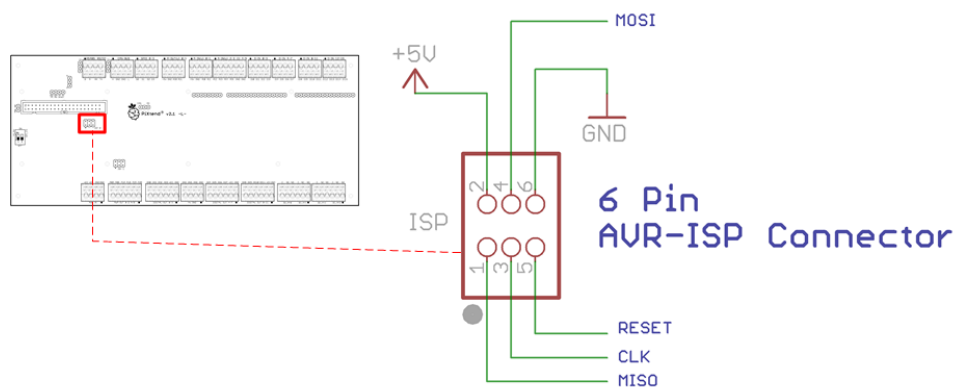
Abbildung 56: Prinzip-Schaltbild: Anschluss eines Programmieradapters an ISP 0 - ATmega324A
